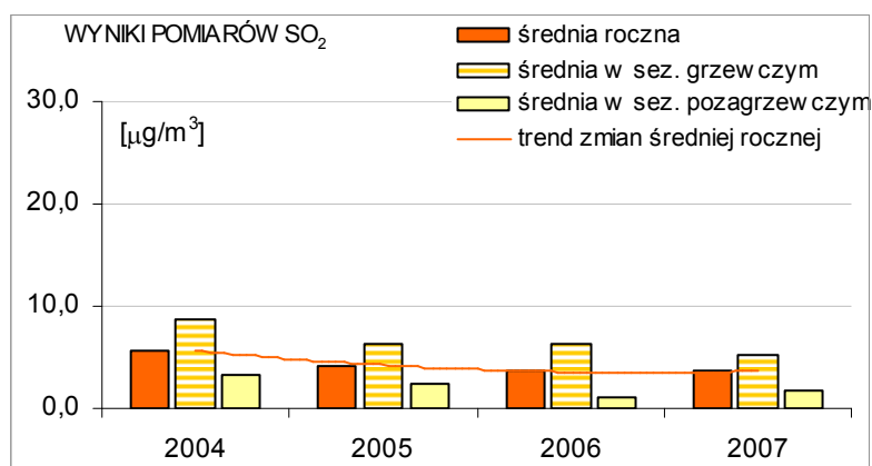
Rysunek 2.23 Wyniki pomiarów dwutlenku siarki [ \mu\text{g}/\text{m}^3 ] (wg WIOŚ).
