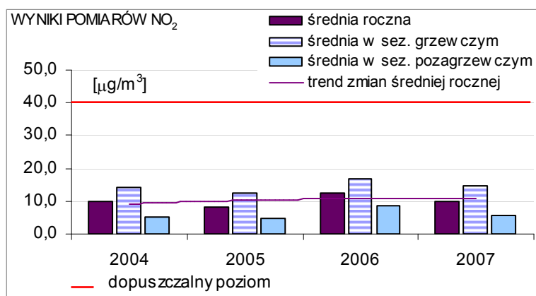
Rysunek 2.24 Wyniki pomiarów dwutlenku azotu [ \mu\text{g}/\text{m}^3 ]
